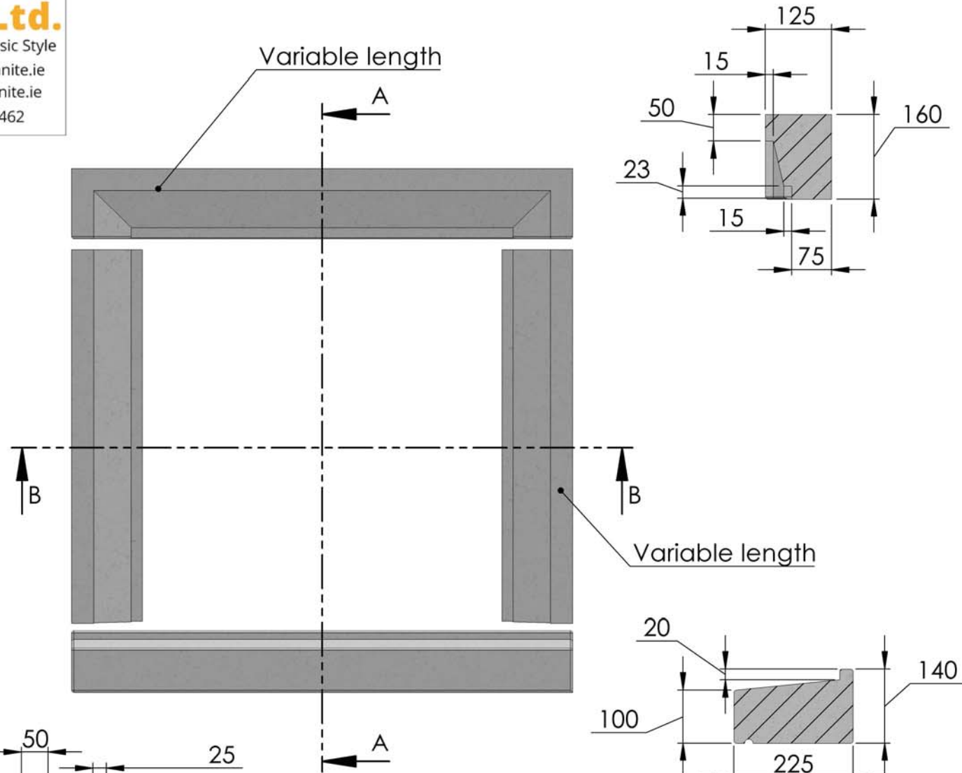
SECTION A-A SCALE 1 : 10
