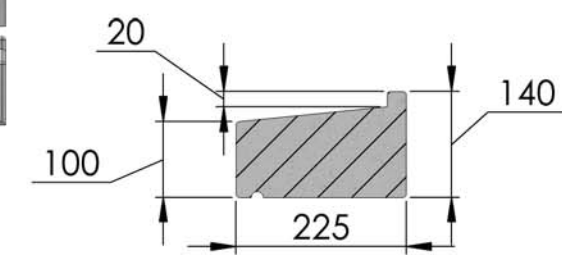
SECTION A-A SCALE 1 : 10
